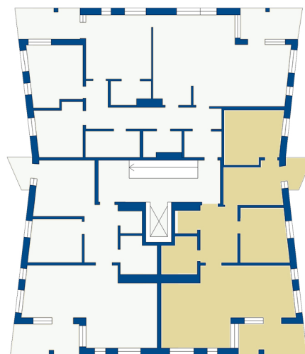
Våningsplan
